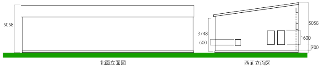
DECO STUDIO Aスタジオ立面图
